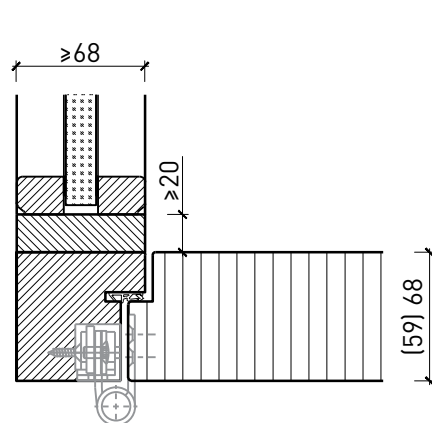
Einbau in Festverglasung mit Glasleisten geschraubt, Türe stumpf
