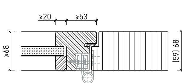
Einbau in Festverglasung mit Glasleisten geschraubt, Türe stumpf
