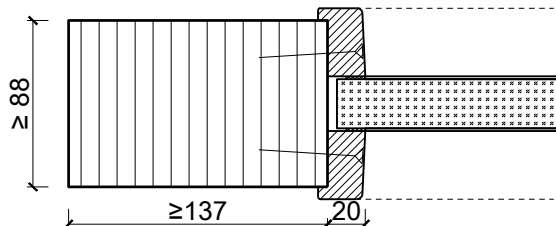
Vitrage centré, parcloses obliques
