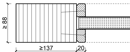
Vitrage centré parcloles droites
