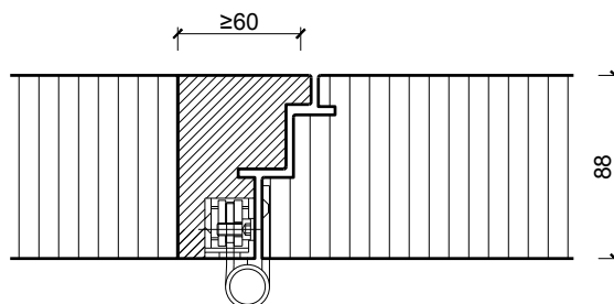
Intégration dans une paroi pleine, porte affleurée
