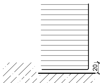
Butée avec joint d'étanchéité 40x30*
