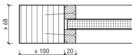
Vitrage centré parcloses droites
