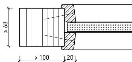
Vitrage centré, parcloses obliques
