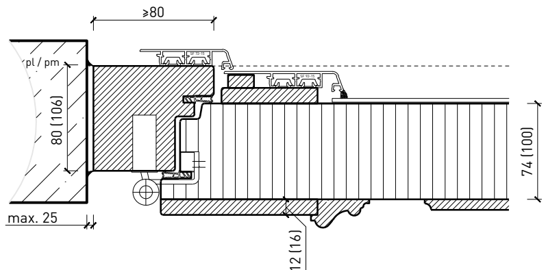
Cadre entre embrasures 74/ 100 mm, porte à battue
