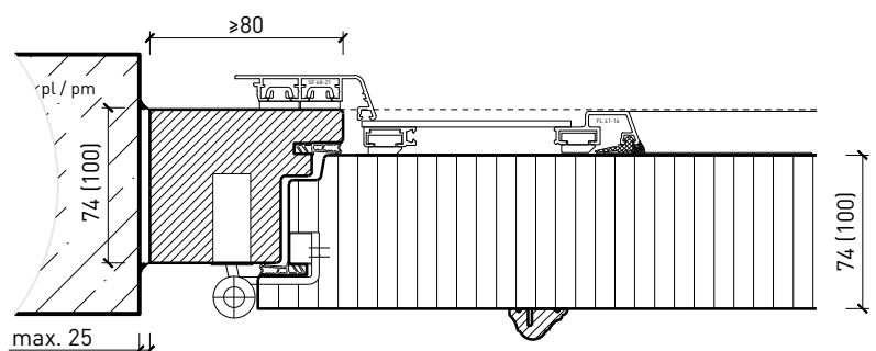
Cadre entre embrasures 74 / 100 mm, porte à battue
