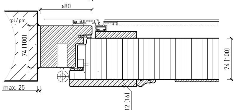
Cadre entre embrasures 74 / 100 mm, porte à battue
