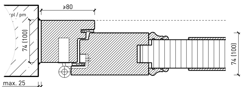
Cadre entre embrasures 74 / 100 mm, porte à battue
