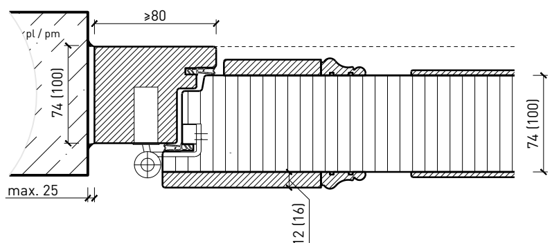
Cadre entre embrasures 74 / 100 mm, porte à battue
