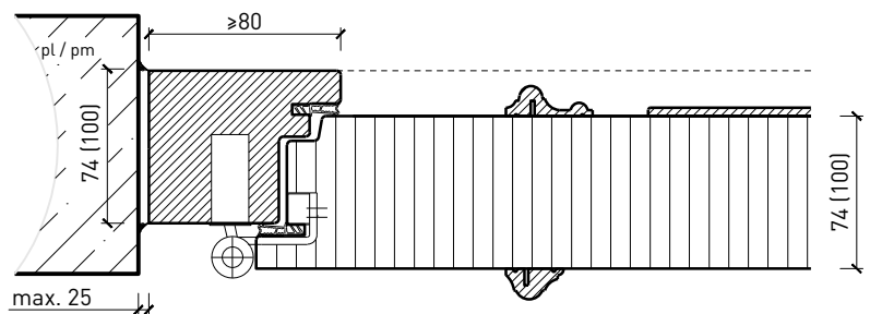
Cadre entre embrasures 74 / 100 mm, porte à battue
