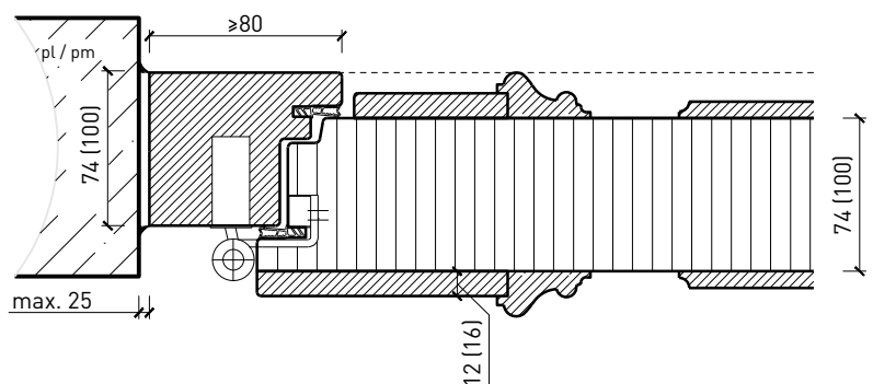
Cadre entre embrasures 74 / 100 mm, porte à battue
