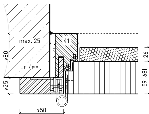
Embrasure de rénovation, porte affleurée avec doublage acoustique
