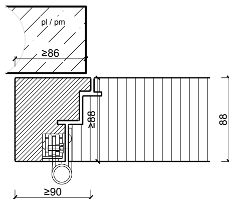
Cadre applique 88 mm, porte affleurée
