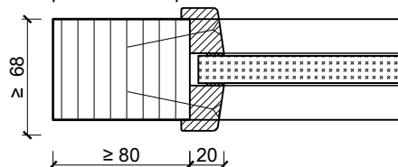
Vitrage centrée, parcloses obliques
