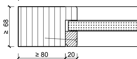
Vitrage centrée parclose d'un côté
