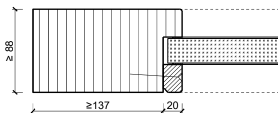
Vitrage centré parclose d'un côté
