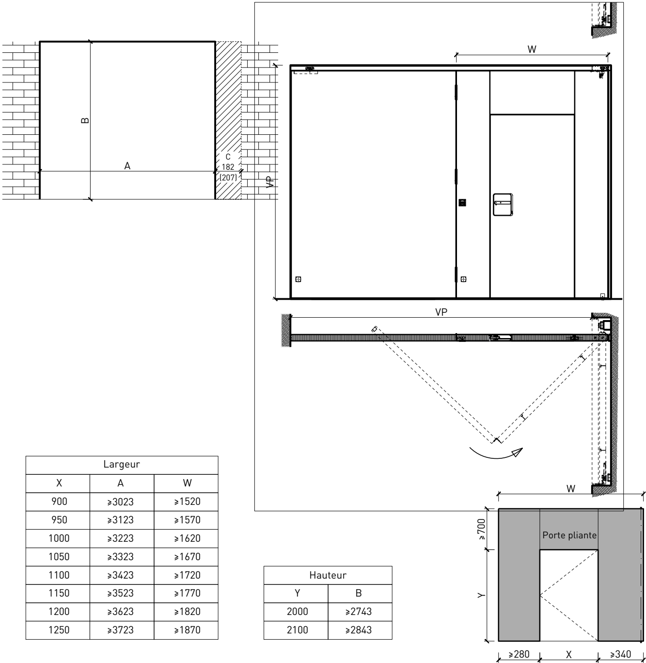
Sense d'ouverture pour des portes de service
