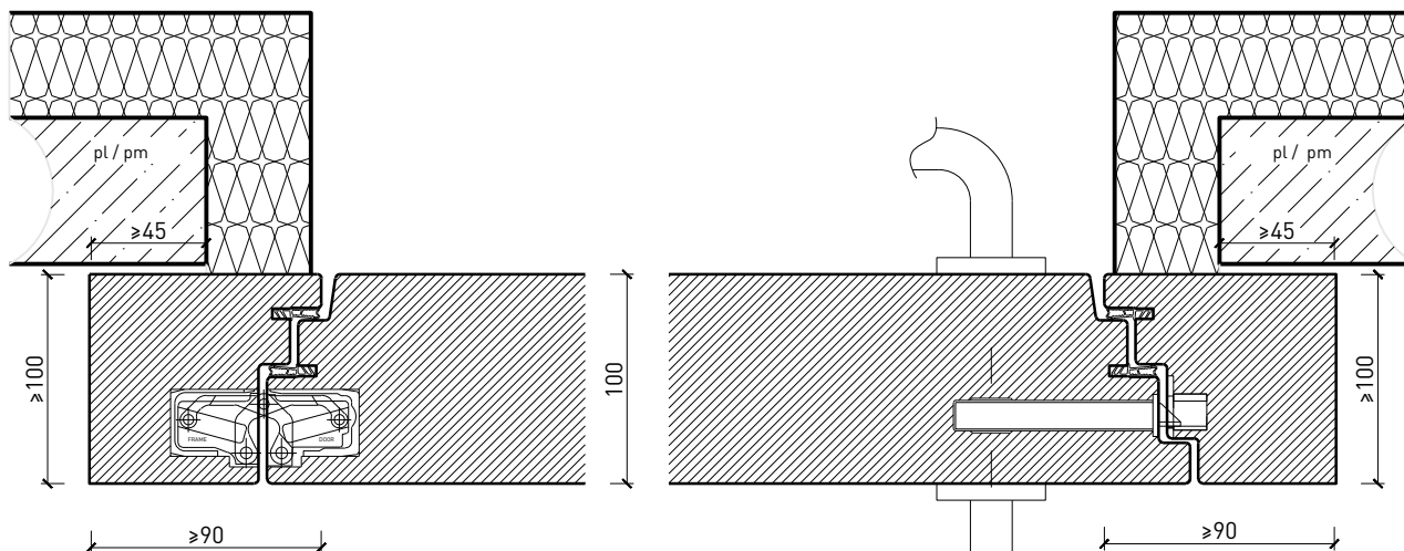
Cadre applique 100 mm, porte affleurée
