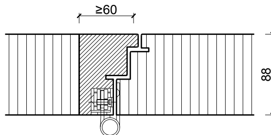
Intégration dans une paroi pleine, porte affleurée
