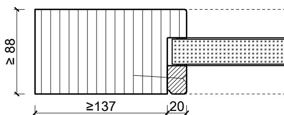
Vitrage centré parclose d'un côté
