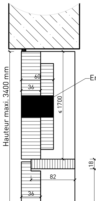
Raccord au plafond avec parement
