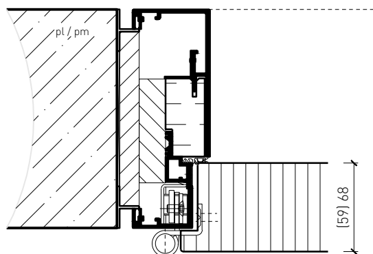
Huisserie en aluminium, porte à battue
