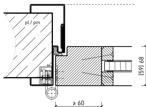
Huisserie enveloppante métallique sans chambrante, porte affleurée
