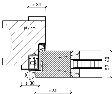
Huisserie enveloppante métallique en deux parties, porte à battue
