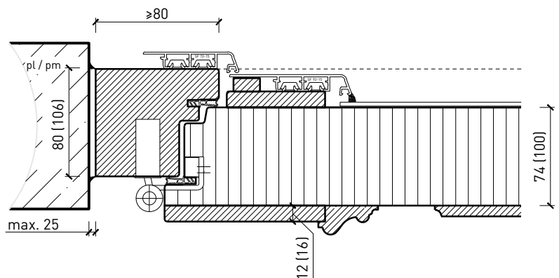
Cadre entre embrasures 74/ 100 mm, porte à battue
