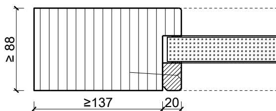
Glas mittig Glasleiste einseitig
