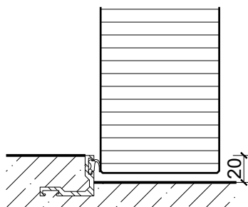
Anschlagwinkel mit Dichtung 40x30*
