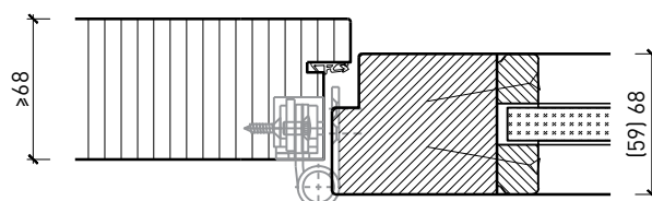
Einbau in Vollwand, Türe stumpf
