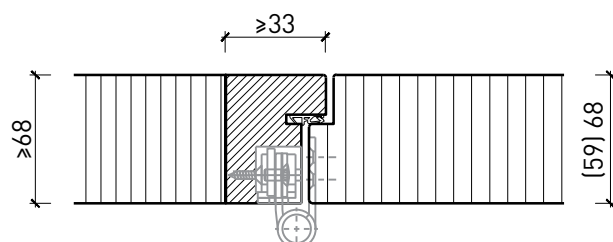
Einbau in Vollwand, Türe stumpf
