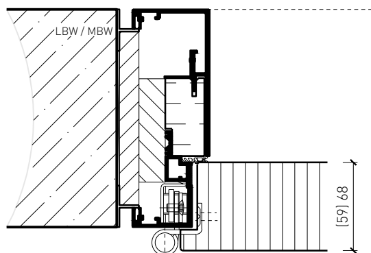
Aluminiumzarge, Türe gefälzt
