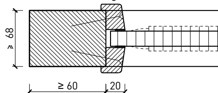
Füllung mittig, Glasleisten schräg
