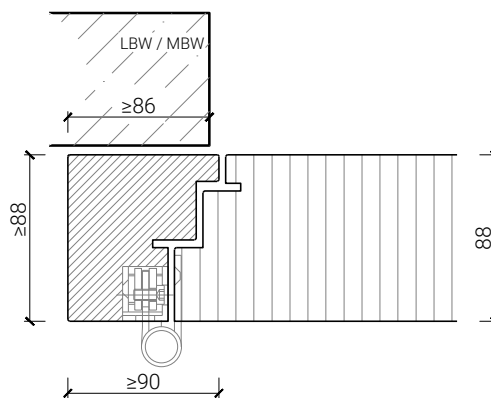
Blendrahmen 88 mm, Türe stumpf
