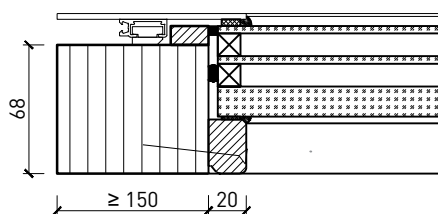
Aluschale glatt Glasleiste schräg
