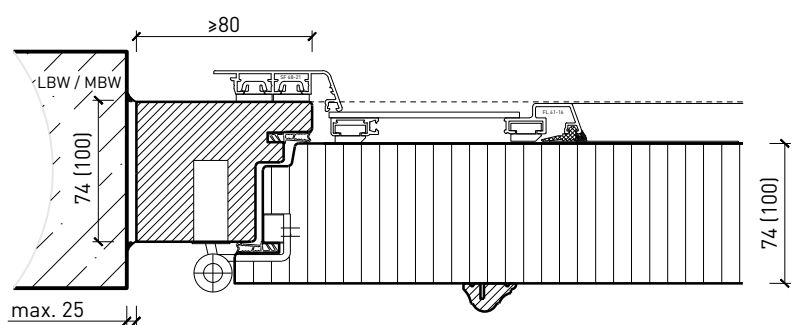
Blockrahmen 74/100 mm, Türe gefälzt
