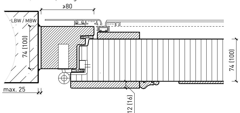
Blockrahmen 74/100 mm, Türe gefälzt
