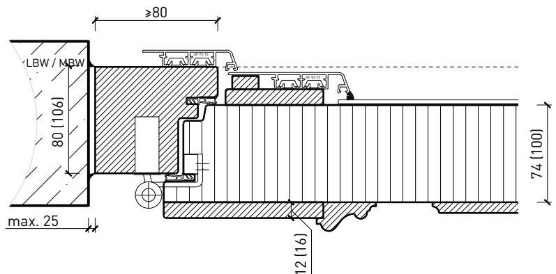
Blockrahmen 80/106 mm, Türe gefälzt
