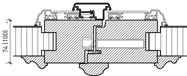
Mittelanschlag 74 / 100 mm, Schlagleisten profiliert
