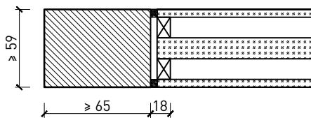
Plano-Verglasung
