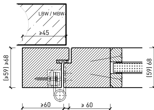
Blockrahmen 59 / 68 mm, Türe stumpf
