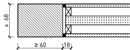
Plano-Verglasung
