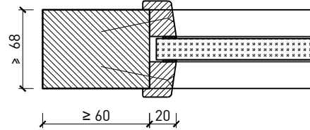
Glas mittig, Glasleisten schräg
