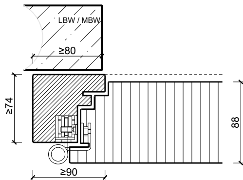
Blendrahmen 74 mm, Türe gefälzt
