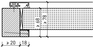
Glas mittig Fensterprofil
