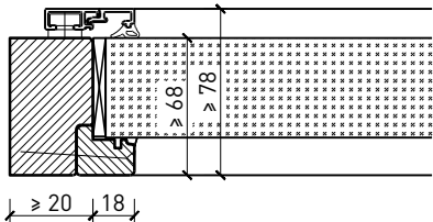
Glas mittig von Aussen eingesetzt
