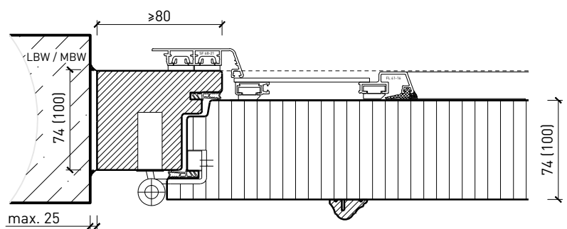
Blockrahmen 74/100 mm, Türe gefälzt
