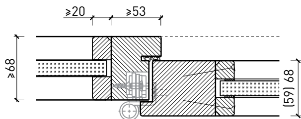
Einbau in Festverglasung mit angefrästen Glasleisten, Türe gefälzt
