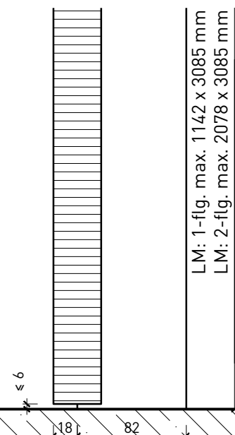
Bodenanschluss schwellenlos
