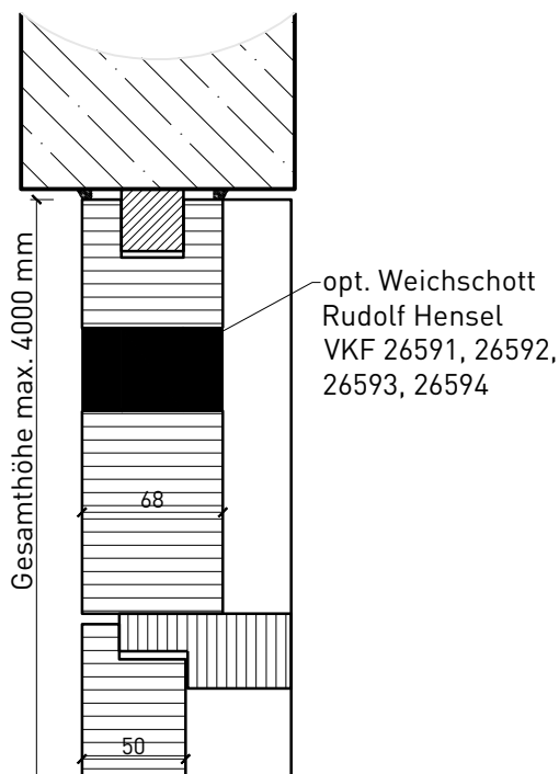
Bodenanschluss schwellenlos
