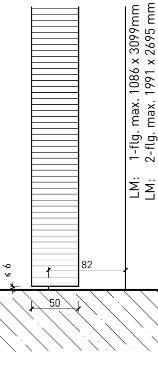
Bodenanschluss schwellenlos
